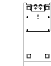
FIGURA 4 FISSAGGIO A PARETE DEGLI ALTOPARLANTI SURROUND
