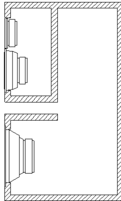
Bassreflex
