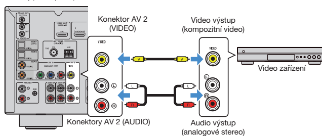
Přístroj (zadní panel)
