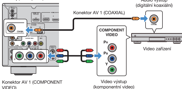
Přístroj (zadní panel)
