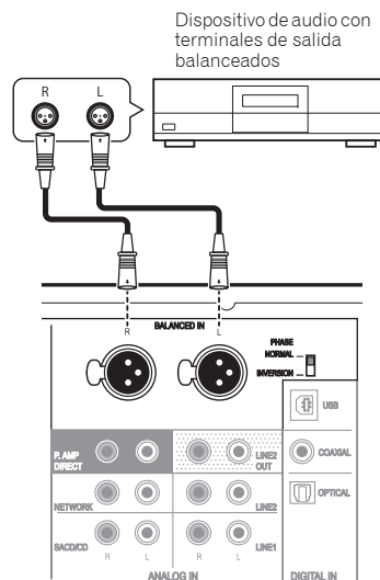
Panel posterior de la unidad A-70DA
