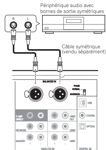
Panneau arrière A-70DA
