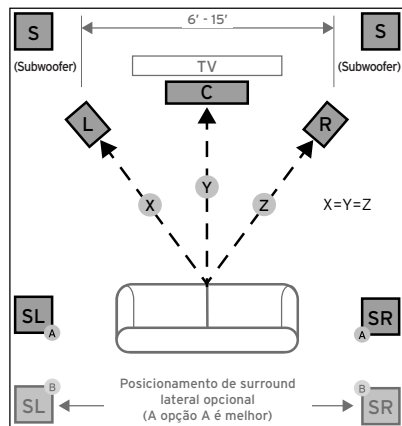
FIGURA 1 POSICIONAMENTO DAS CAIXAS ACÚSTICAS NO AMBIENTE
