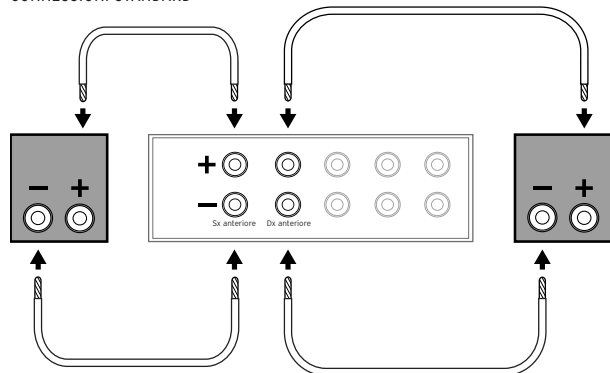
FIGURA 3 CONNESSIONI STANDARD
