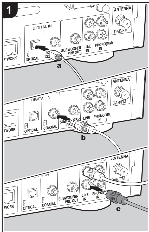
a Digitales optisches Kabel, b Digitales Koaxialkabel, c Analoges Audiokabel
