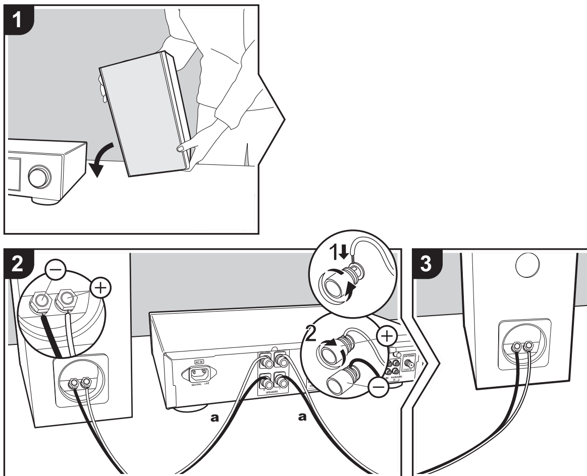
a Cavi dei diffusori
