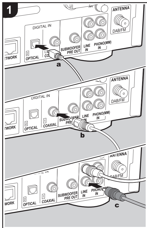
a Cavo digitale ottico, b Cavo digitale coassiale, c Cavo audio analogico
