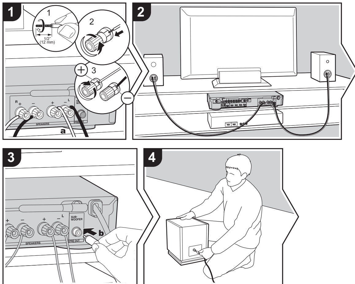
a Högtalarkabel, b Subwooferkabel
