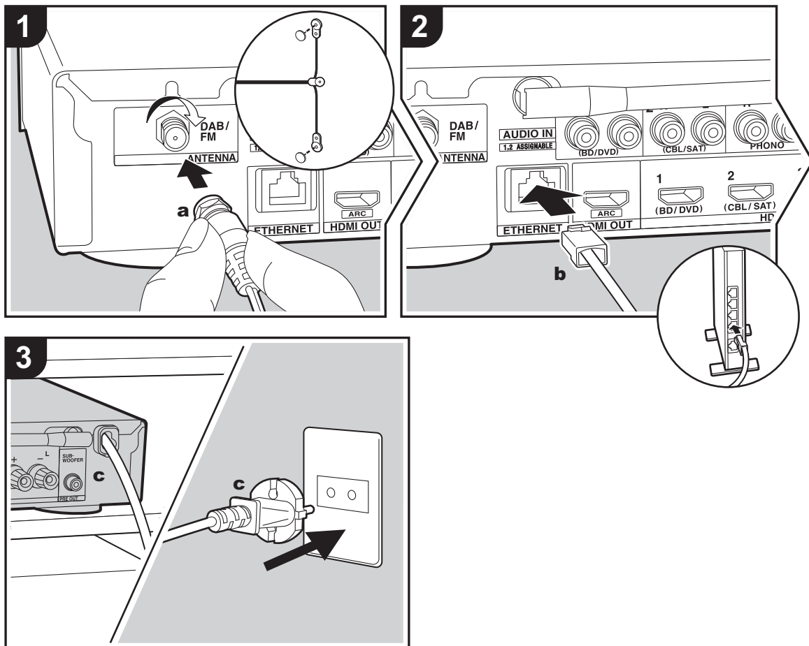
a DAB/FM-antenn, b Ethernet-kabel, c Nätkabel
