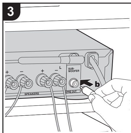
a Cable de altavoz, b Cable de subwoofer
