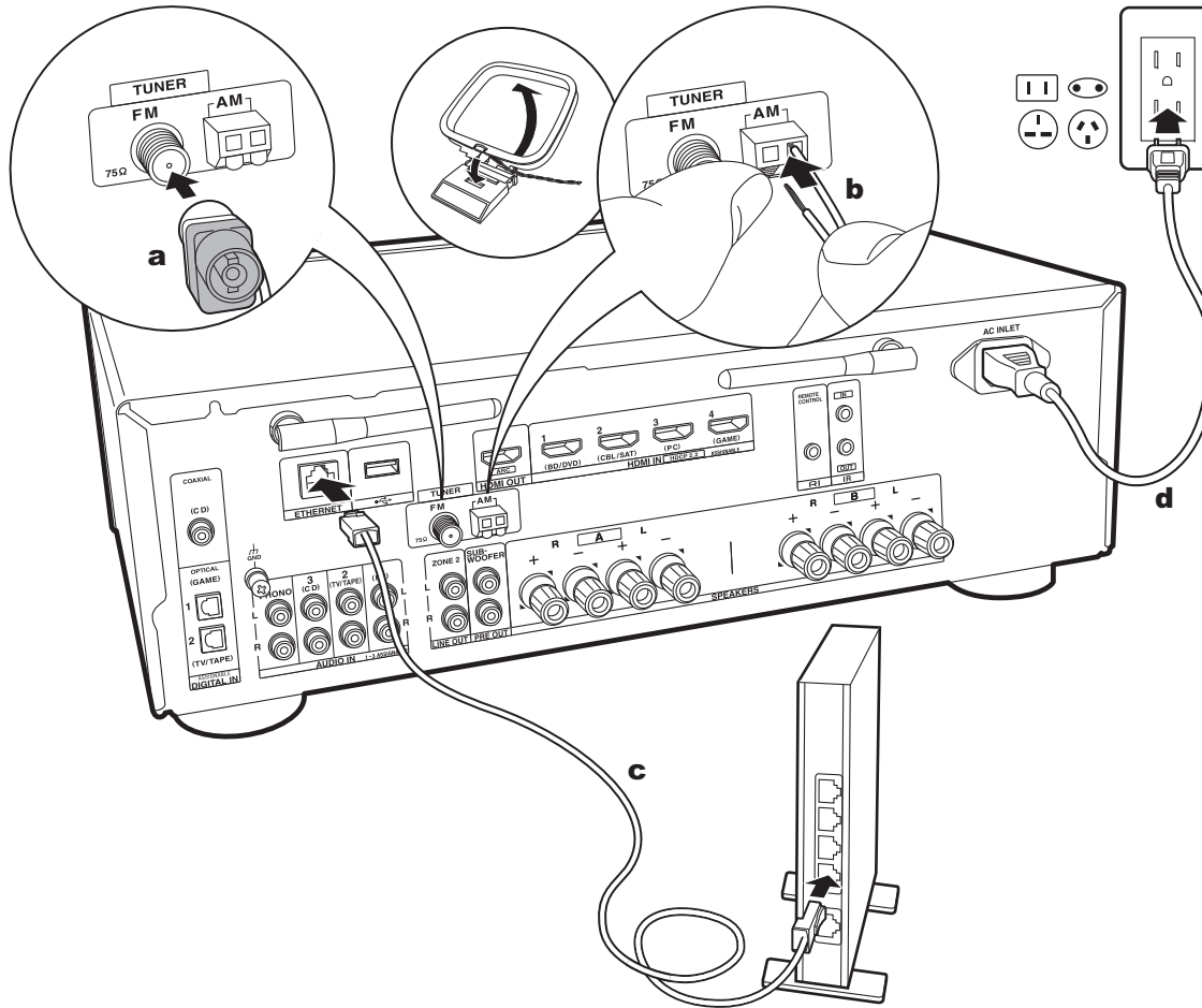
a Antena FM para interiores, b Antena AM para interiores, c Cable Ethernet, d Cable de
